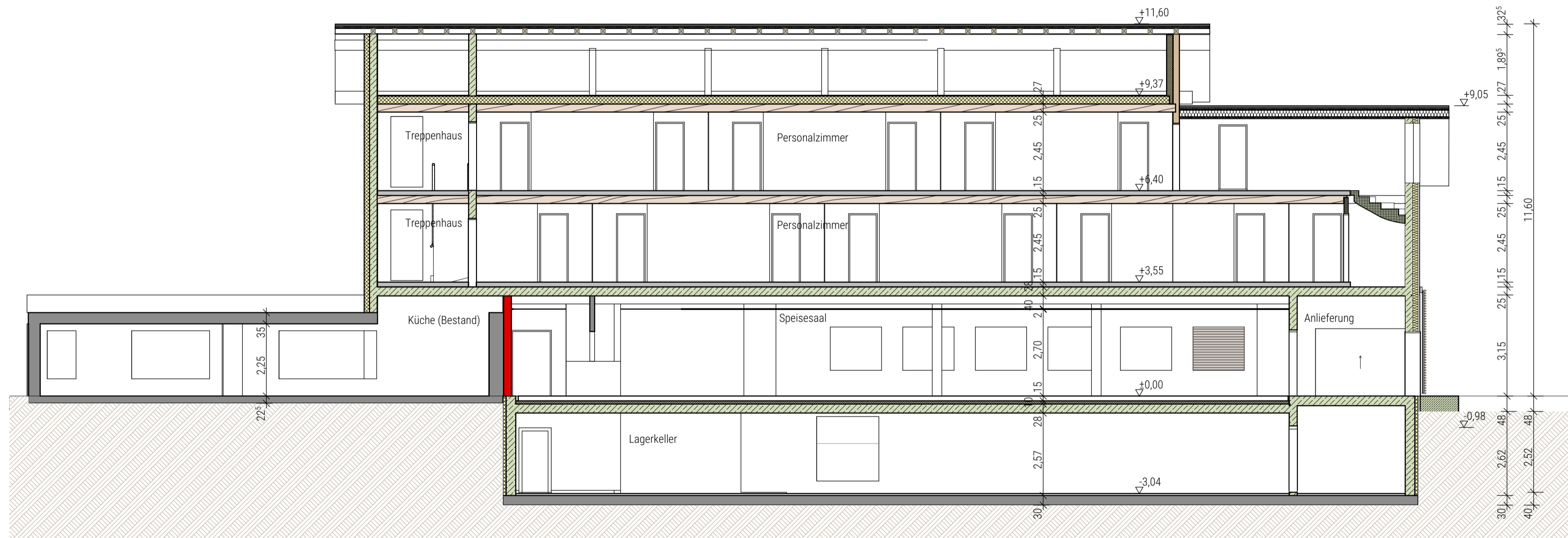
Schnitt A-A
